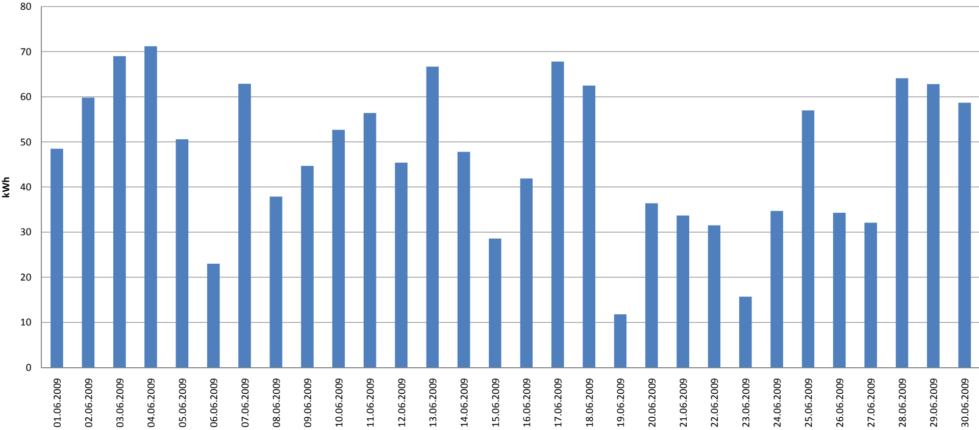
Leistung der Photovoltaikanlage www.posthof.ch im Juni 2009 (Total: 1410.20 kWh)
